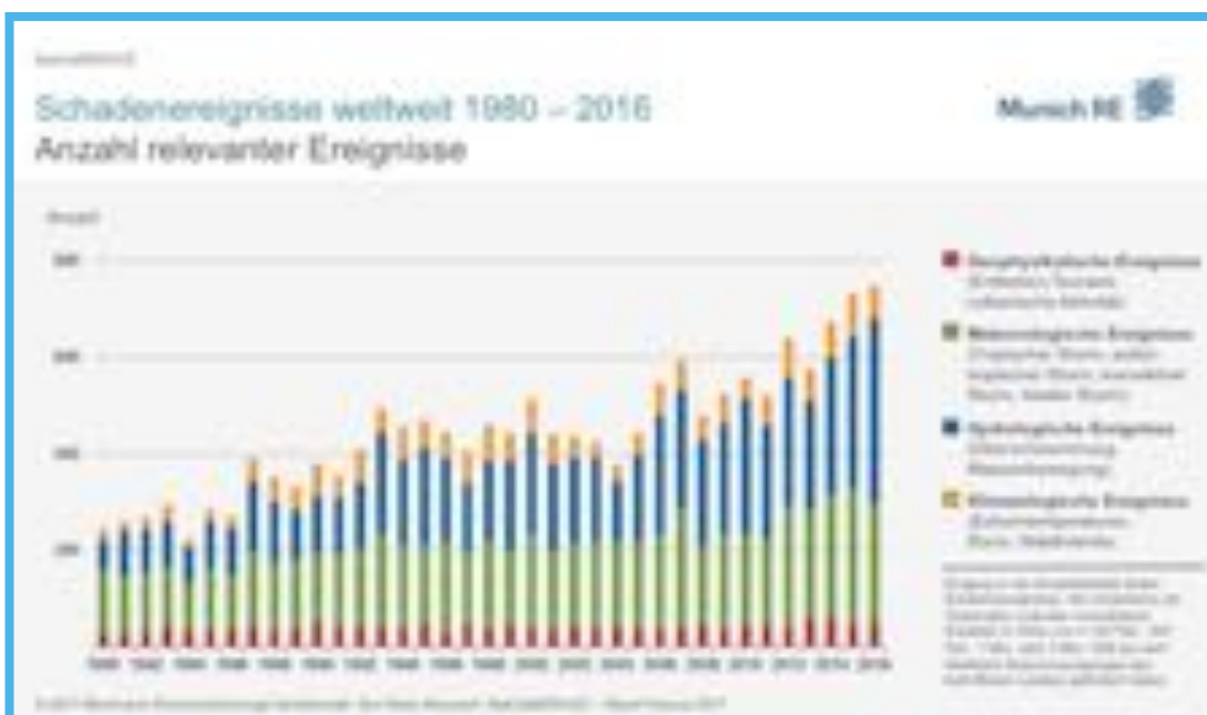
Abb. 1: Schadenereignisse weltweit 1980 – 2016, Anzahl relevanter Ereignisse, Münchner Rück, Februar 2017
