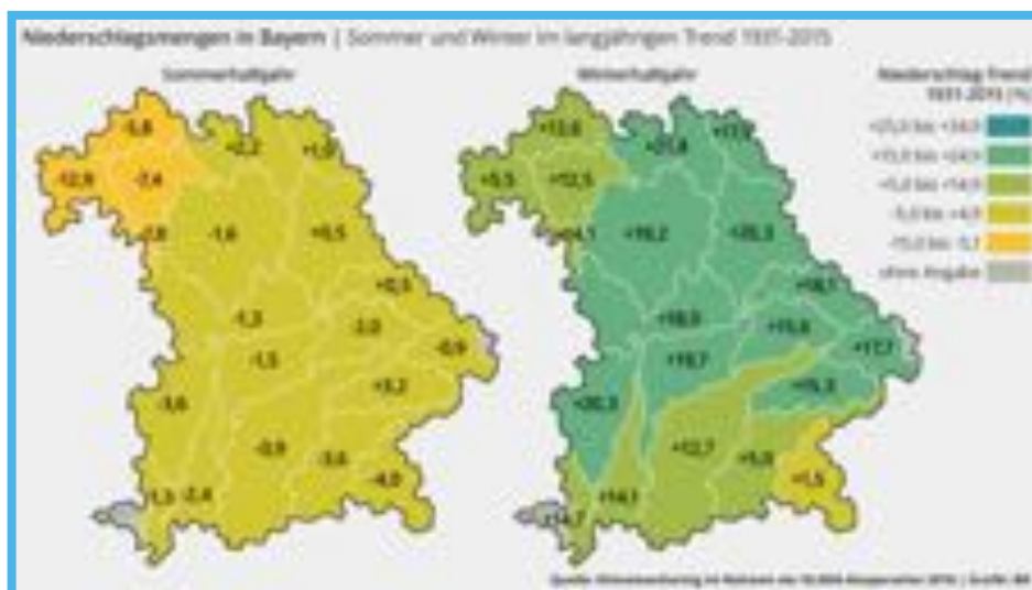
Abb. 7: Langjähriger Trend der Niederschlagsmengen in den Regionen Bayerns 16
