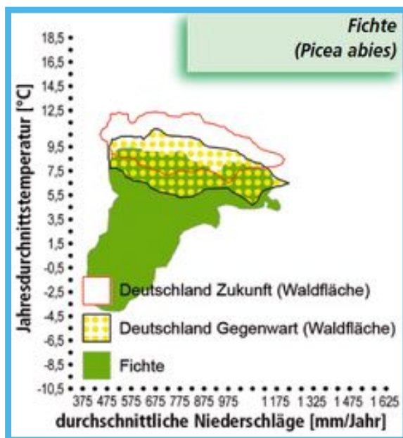
Abb. 18: Baumarten im Vergleich von 2000 zu 2010 (Klimaszenario A1B) abgeleitet aus Nischenmodellen Quelle: Umweltbundesamt 46
