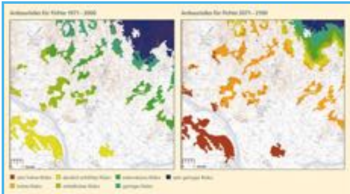
Abb. 17: Anbaurisiko der Fichte mit den Klimawerten der Perioden 1971-2000 und 2071-2100. Klimamodell WETTREG, Szenario B1, Der Kartenausschnitt zeigt das Donautal bei Irlbach und den Anstieg zum Bayerischen Wald. (Quelle: LWF, Daten: LfU, Bayer. Vermessungsverwaltung, DWD)
