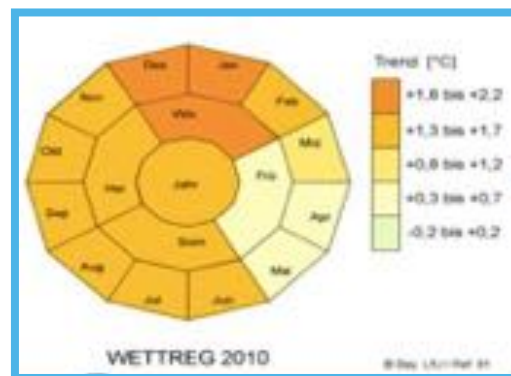
Abb. 5: Änderungssignal der Mitteltemperatur in Bayern von 2021-2050 gegenüber 1971-2000 10
