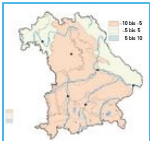
Abb. 9: Projizierte relative Änderung [%] der Grundwasserneubildung in der nahen Zukunft (2021–2050) innerhalb der Naturräume Bayerns anhand der Projektion WETTREG2006 21
